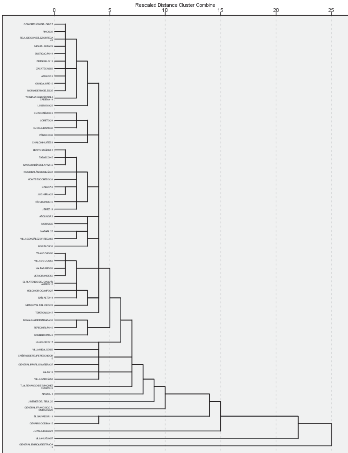
Grafica 1. Dendograma
